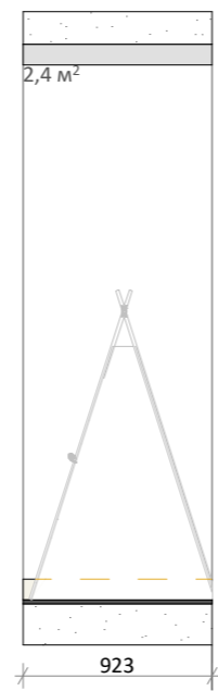
2-2 1:40
