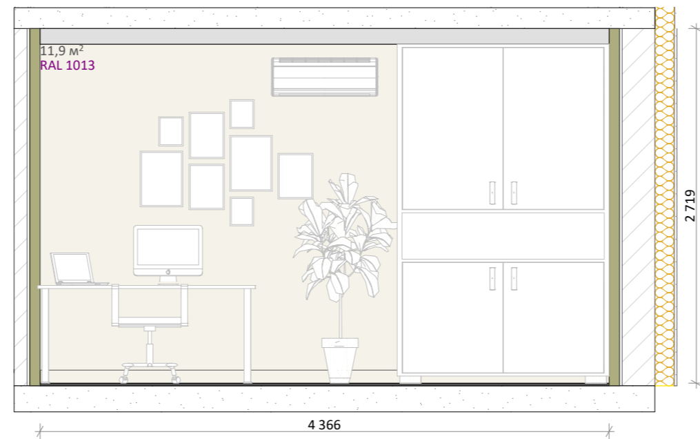
2-2 1:40
